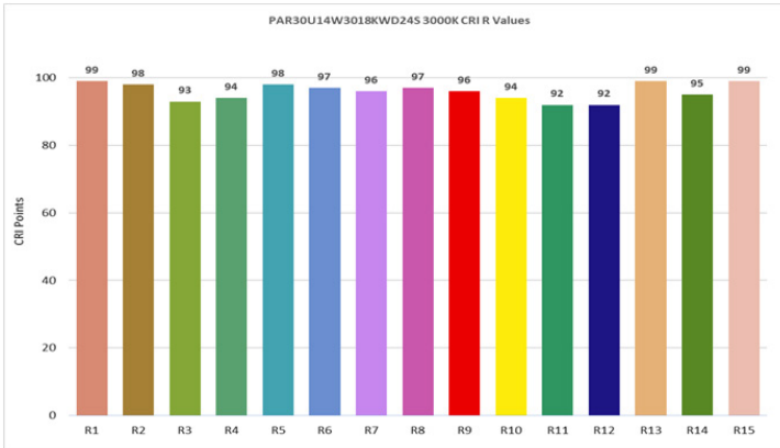
3000K (220V)
